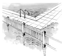
Fixação de cercas a enterrar no solo
