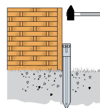
Fixação de cercas a enterrar no solo
