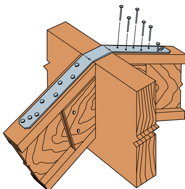
Fita de aço LSTA instalado com N3.75
