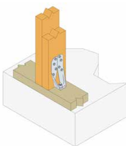
Ancoragem longitudinal DTT instalado com SDS
